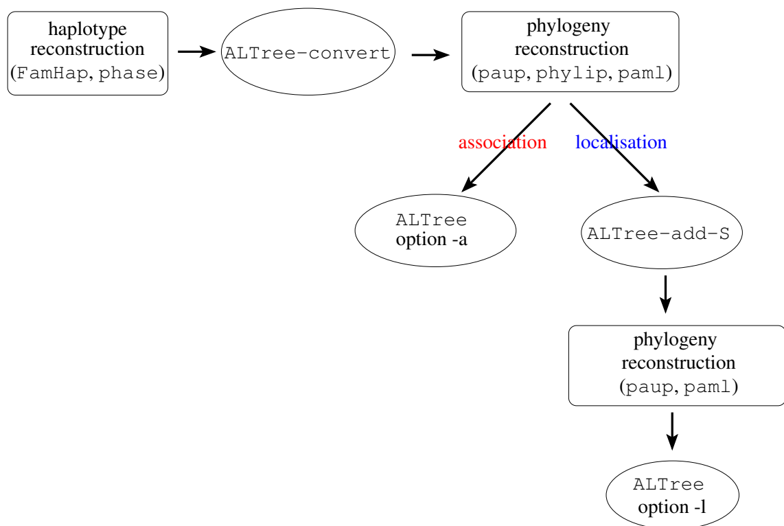
Figure I: ALTree programs
